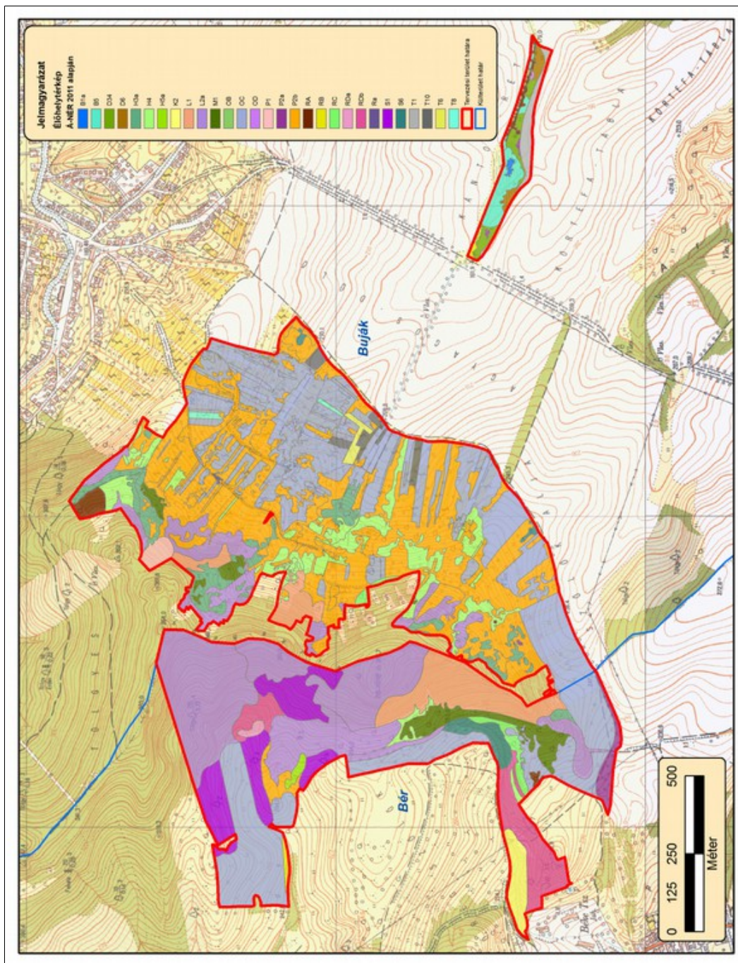
6. ábra: A tervezési terület élőhelytérképe. (B1a - Nem tőzegképző nádasok, gyékényesek és tavikákások; B5 - Nem zsombékoló magassárrétek; D34 – Mocsárrétek; D6 - Artéri és mocsári magaskórósok, árnyas-nyirkos szegélynövényzet; H3a - Köves talajú lejtősztyepek; H4 - Félszáraz irtásrétek, száraz magaskórósok és erdőssztyeprétek; H5a - Lőszgyepek, kötött talajú sztyeprétek; L2a - Cseres-kocsánytalan tölgyesek; K2 - Gyertyános-kocsánytalan tölgyesek; M1 - Molyhos tölgyes bokorerdők; OB - Jellegtelen üde gyepek és magaskórósok; OC - Jellegtelen száraz-félszáraz gyepek; OD - Lágyszárú özönfajok állományai; P1 - Őshonos fajú fiatalosok; P2a - Üde és nedves cserjések; P2b – Galagonyás-kökényes-borókás cserjések; RA - Őshonos fajú facsoportok, fasorok, erdősavok; RB - Puhafás pionír és jellegtelen erdők; RC - Őshonos fajú keményfás pionír és jellegtelen erdők; RDa - Őshonos lombos fajokkal elegyes fenyves származékerdők; RDb - Őshonos lombos fajokkal elegyes idegenhonos lombos és vegyes erdők; S1 - Akác ültetvények; S6 - Nem őshonos fajok spontán állományai; T1 - Egyéves, nagyüzemi szántóföldi kultúrák; T6 - Extenzív szántók; T8 - Extenzív szőlők és gyümölcsösök; T10 - Fiatal parlag és ugar)
